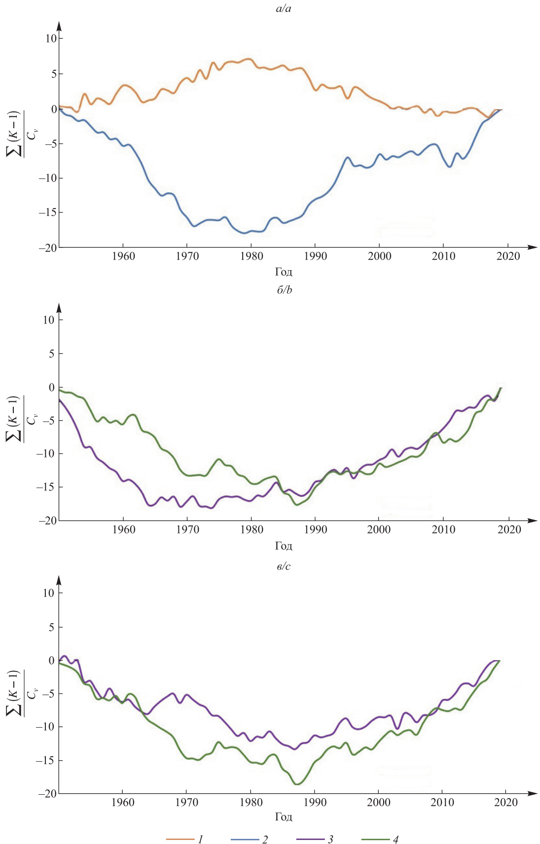
Рис. 2. Разностные интегральные кривые: a – индексы атмосферной циркуляции SCAND (1) и NAO (2); b , в – суммарные осадки (3) и приземная температура воздуха (4) для северной и южной частей региона соответственно
