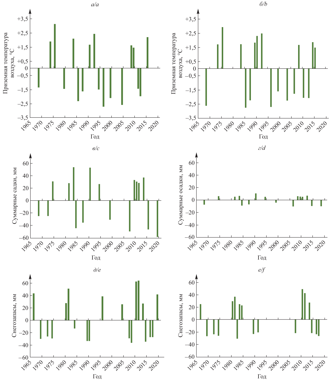
Рис. 3. Многолетний ход аномалий (превышение стандартного отклонения) снегозапасов, приземной температуры воздуха и суммарных осадков в северной ( a, в, д ) и южной ( б, г, е ) частях региона
