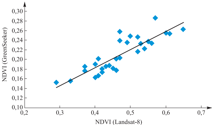
Рис. 5. Диаграмма рассеяния значений индекса NDVI, полученных наземными (GreenSeeker) и спутниковыми (Landsat-8) методами
