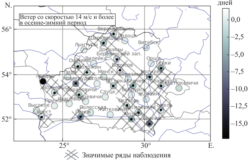
Рис. 18. Карта распределения числа дней с ветром со скоростью 14 м/с и более на территории Беларуси в осенне-зимний период за 1975–2021 гг.
