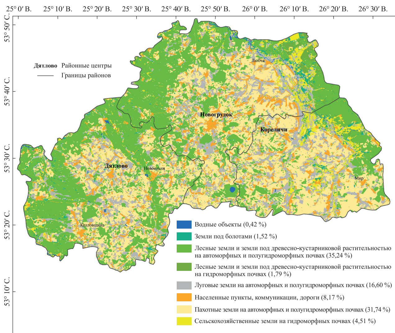
Рис. 2. Структура земельного покрытия Новогрудской возвышенности в 1986 г. на основе космического снимка «Landsat-5».
