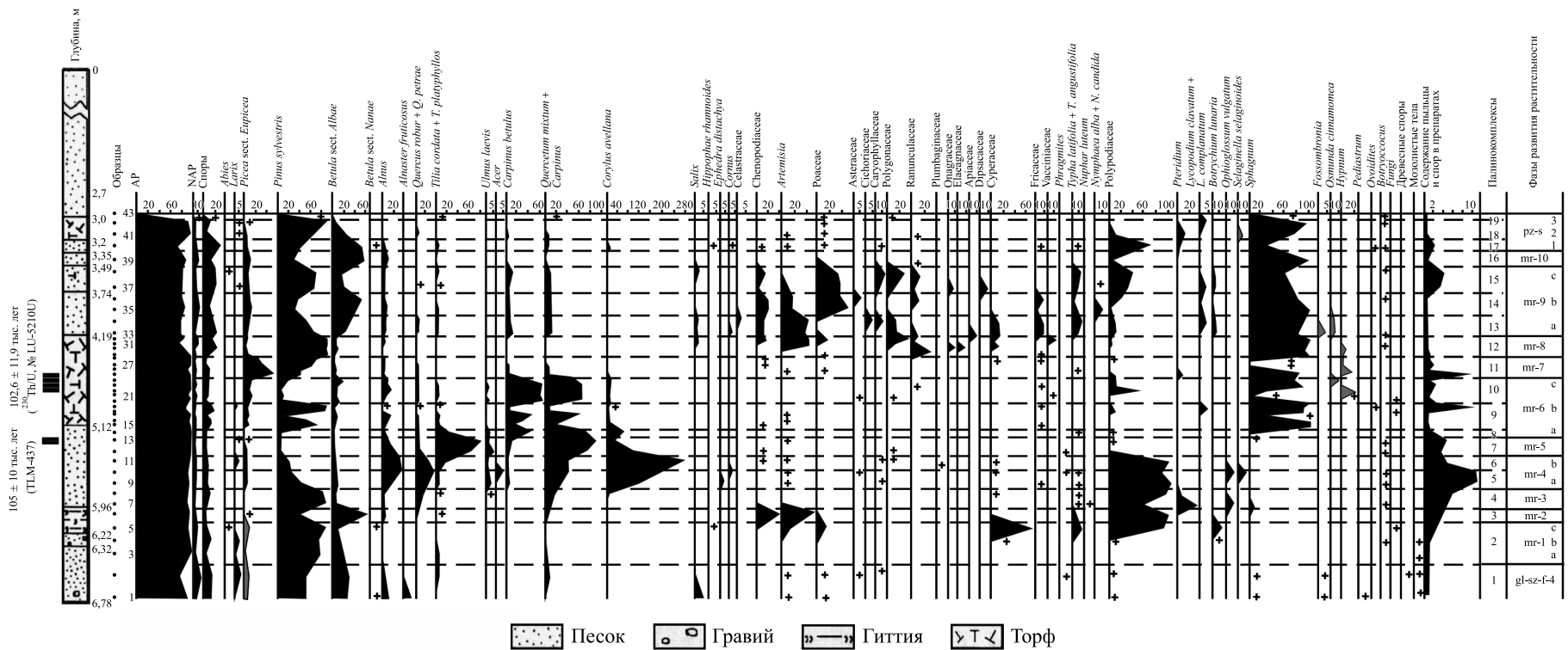
Рис. 2. Палинологическая диаграмма древнеозерных отложений у д. Муравы
