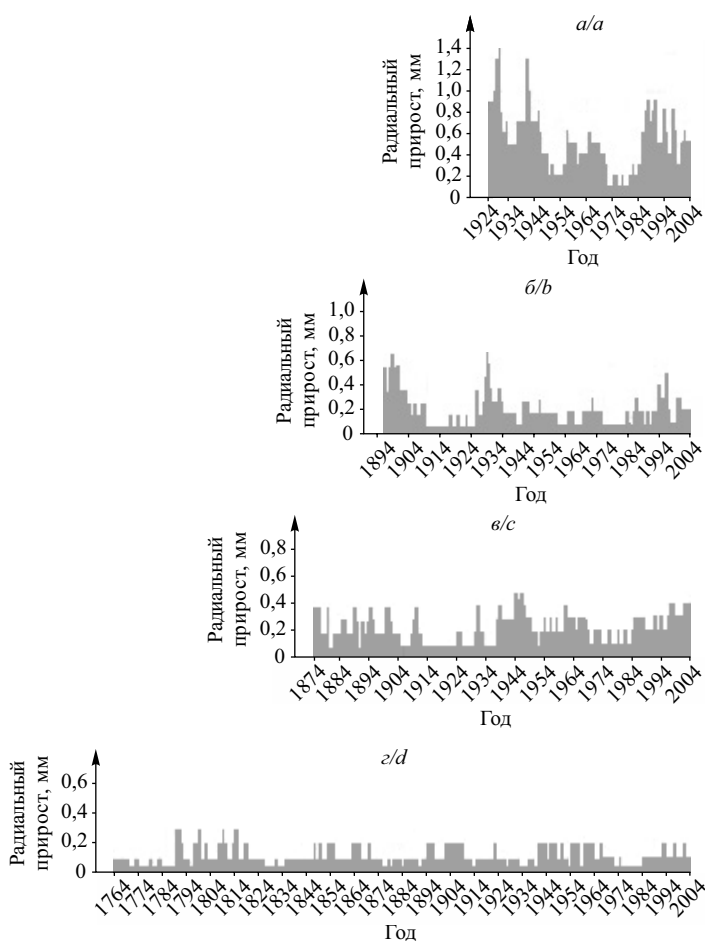
Рис. 1. Многолетний погодичный ход изменчивости минимального индивидуального радиального прироста возрастных серий сосны на территории верхового болота Круки: a – 85 лет; б – 115 лет; в – 140 лет; г – 250 лет
