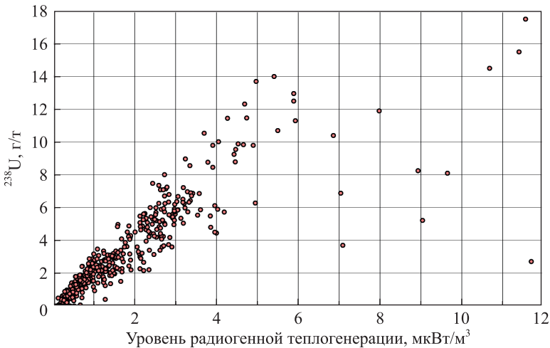
Рис. 5. Связь значений концентрации изотопа ^{238}\text{U} с уровнем радиогенной теплогенерации
