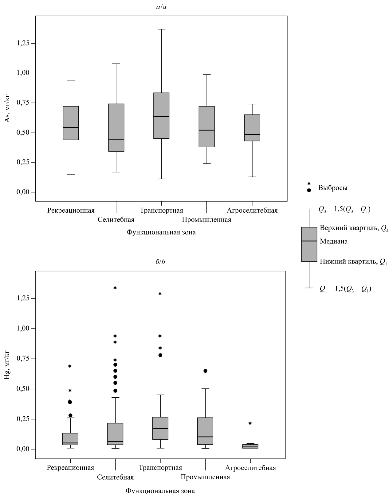
Рис. 2. Параметры варьирования содержания As (а) и Hg (б) в землях (почвах) (0–20 см) различных функциональных зон урбанизированных территорий Беларуси
