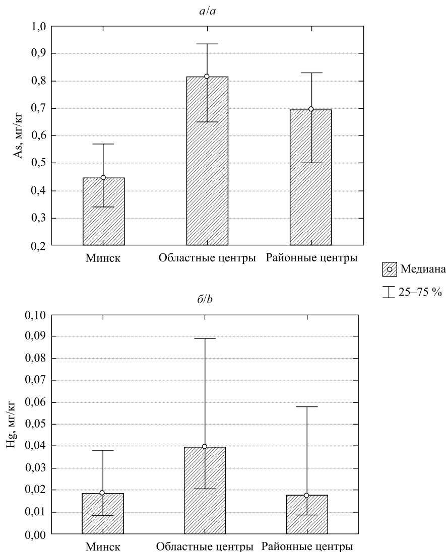
Рис. 5. Диаграмма содержания As (а) и Hg (б) в землях (почвах) (0–20 см) г. Минска, областных и районных центров Fig. 5. Diagram of As (a) and Hg (b) content in lands (soils) (0–20 cm) within Minsk, regional and district centres
