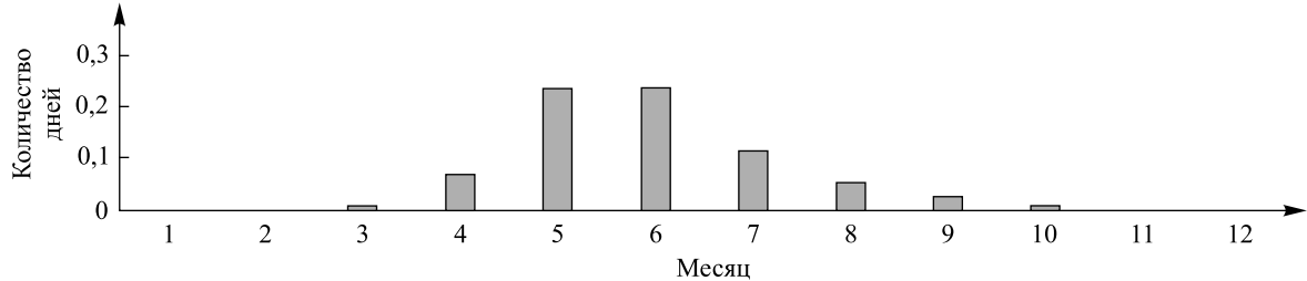
Рис. 6. Хронологический ход многолетнего среднемесячного количества дней с градом за 1989–2016 гг.
