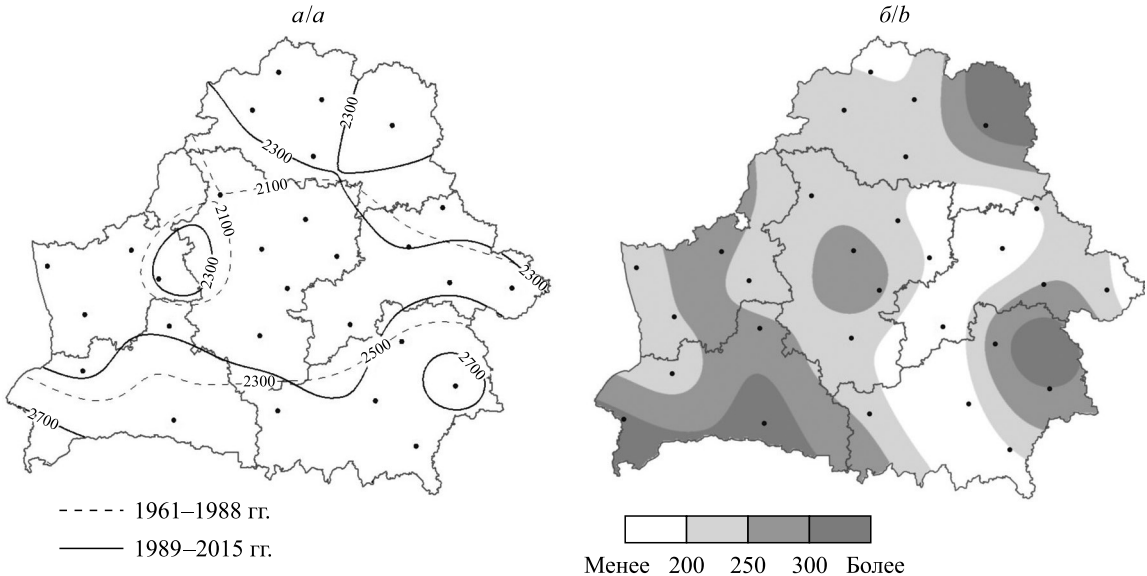
Рис. 2. Суммы активных температур выше 10 °С ( а ) и их прирост ( б ) в 1989–2015 гг. по сравнению с 1961–1988 гг.
