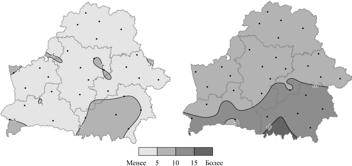
Рис. 5. Количество дней с максимальной температурой воздуха выше 30 °С в годы наличия за 1961–1988 гг. (а) и 1989–2015 гг. (б)
