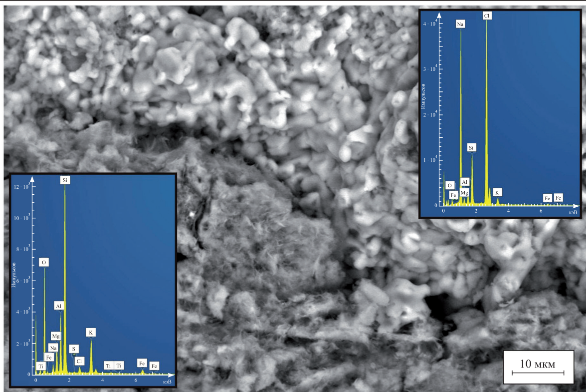
Рис. 4. Микрофотографии SEM и спектры EDX туфа (светлый участок – галит, темный – иллит)
