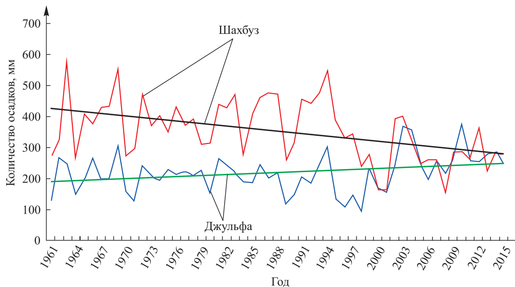
Рис. 4. Многолетняя динамика и тенденции изменения количества атмосферных осадков по гидрометеорологическим станциям Джульфы и Шахбюз
