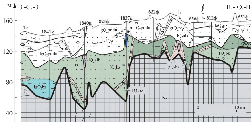
Рис. 5. Строение Малоритской ложбины и флювиогляциального конуса выноса на ее дистальном окончании (а – план поверхности березинского ледникового горизонта; б – продольный разрез по линии аг. Страдечь Брестского района – аг. Хотислав Малоритского района; в – поперечный разрез по линии д. Язвин – д. Богуславка Малоритского района). Условные обозначения см. на рис. 3
