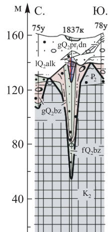
Рис. 5. Строение Малоритской ложбины и флювиогляциального конуса выноса на ее дистальном окончании (а – план поверхности березинского ледникового горизонта; б – продольный разрез по линии аг. Страдечь Брестского района – аг. Хотислав Малоритского района; в – поперечный разрез по линии д. Язвин – д. Богуславка Малоритского района). Условные обозначения см. на рис. 3
