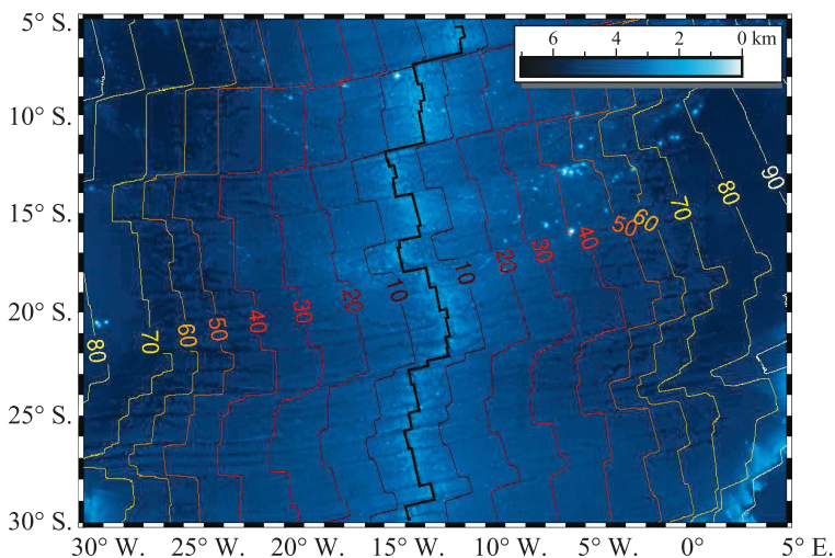
Рис. 9. Связь между возрастом и мощностью океанической коры
