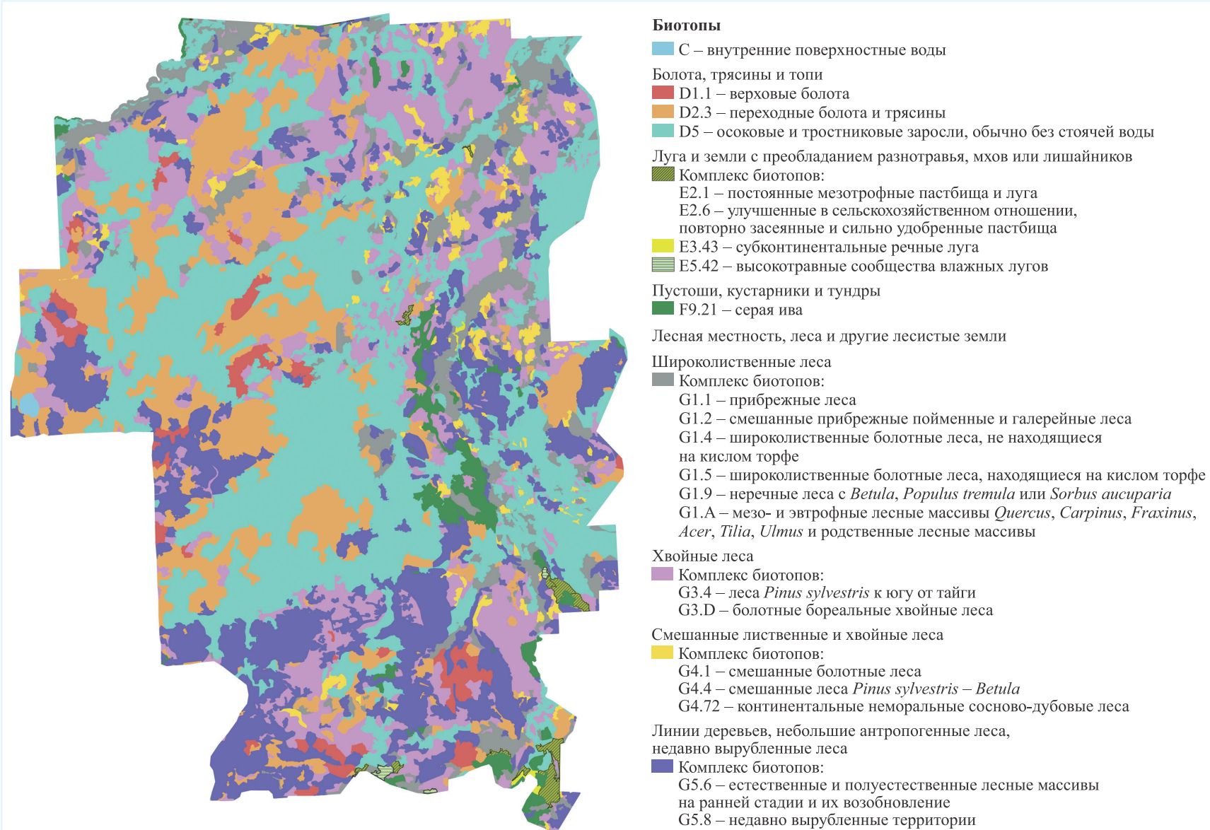
Рис. 3. Биотопы ВБУ «Ольманские болота», выявленные на основе классификации EUNIS
