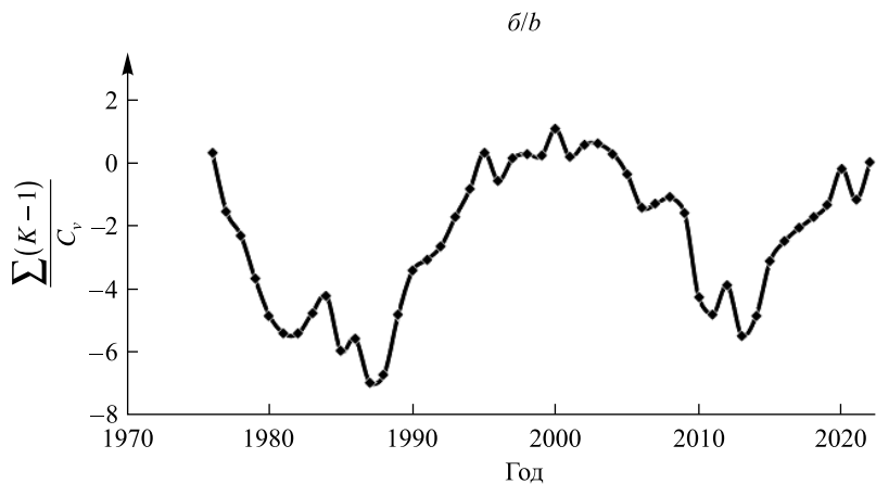
Рис. 5. Интегральные кривые индексов арктической (а) и североатлантической (б) осцилляций
