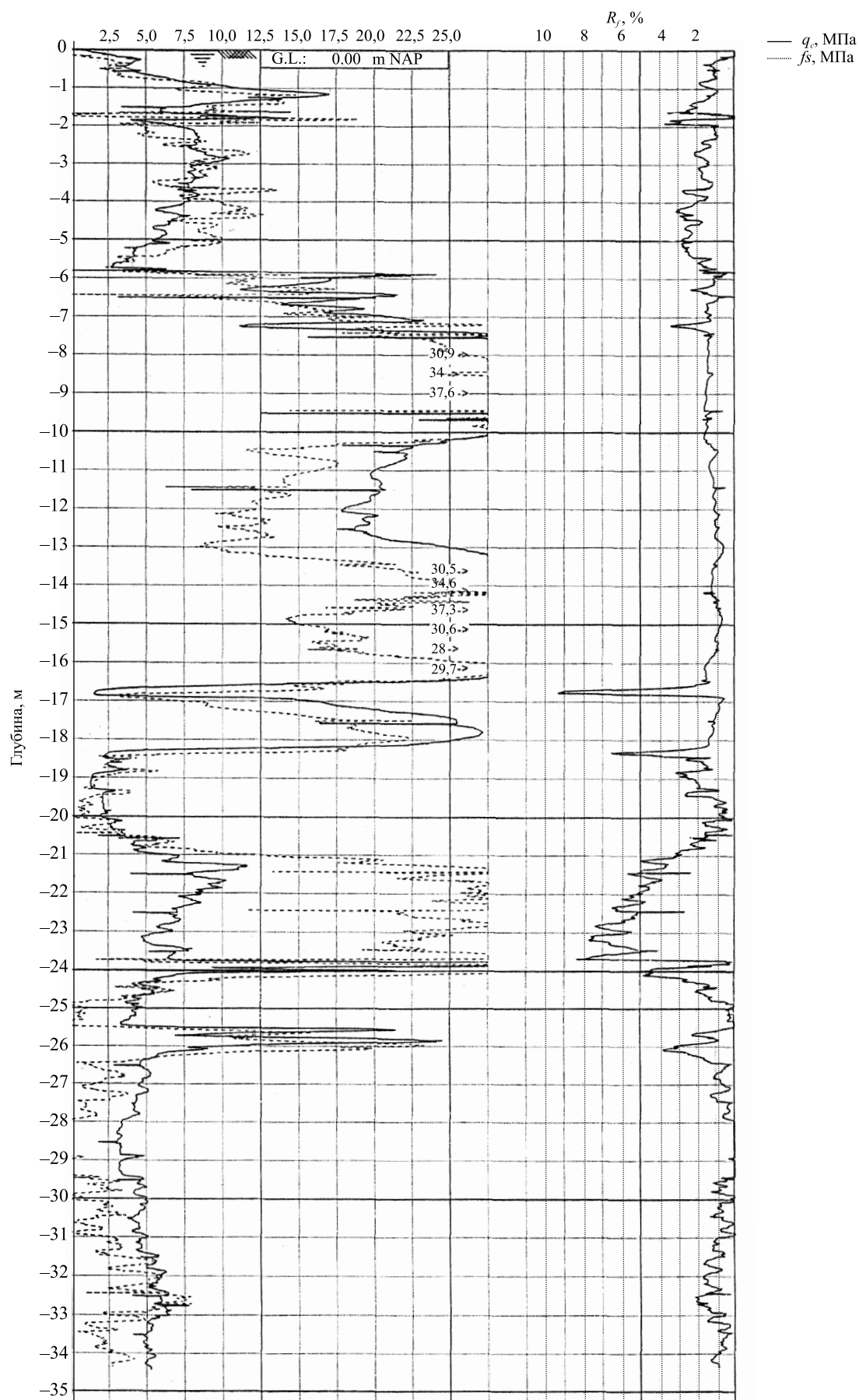
Рис. 4. Точка глубокого статического зондирования (по материалам изысканий УП «Геосервис»)
