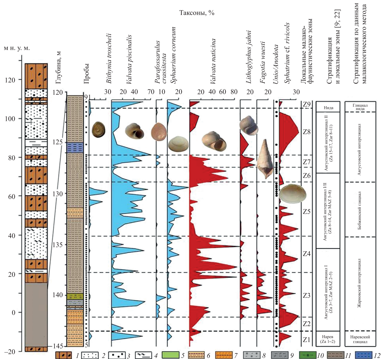
Рис. 4. Малакологическая диаграмма отложений, вскрытых скважиной Жарново на северо-востоке Польши:
