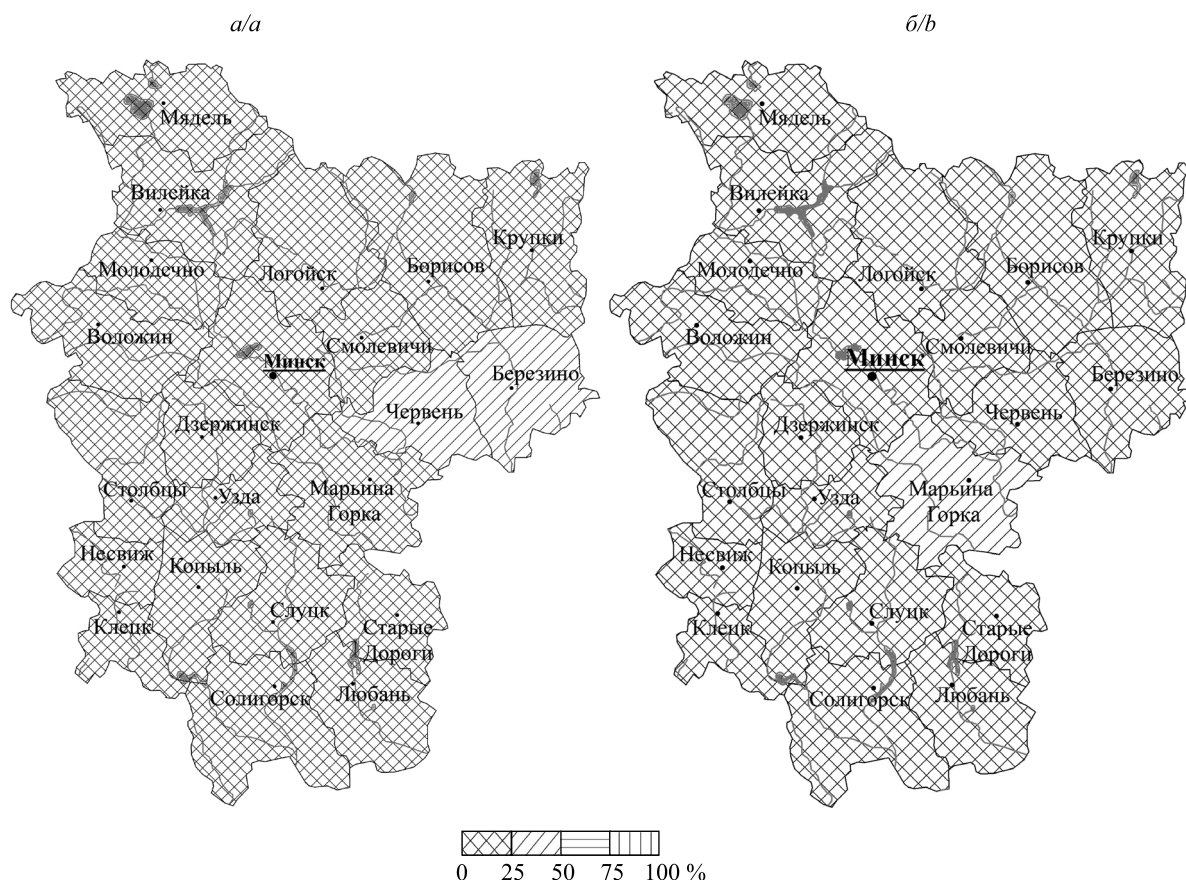
Рис. 1. Доля пригодных участков рек Минской области для контактных видов туризма и отдыха: а – купания; б – подводного плавания
