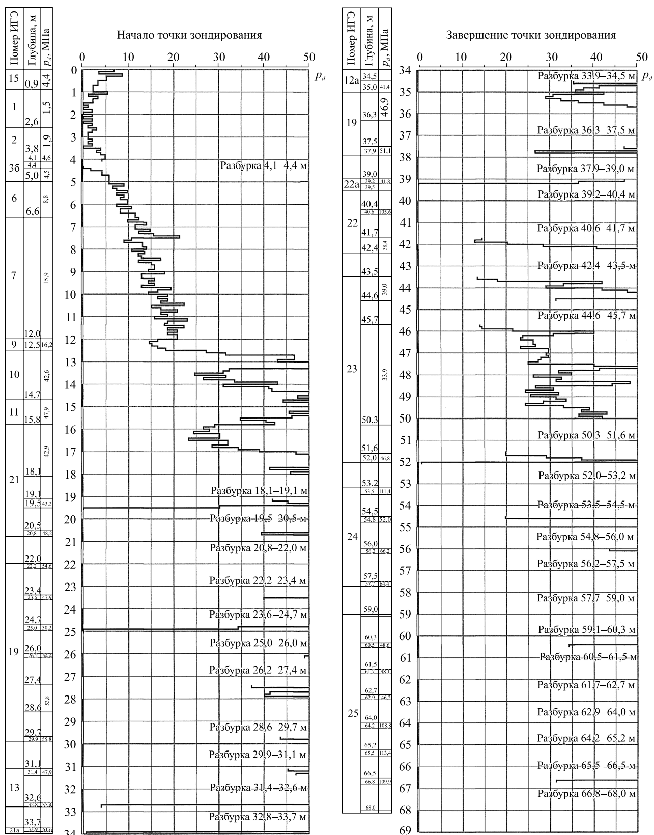
Рис. 3. Точка глубокого динамического зондирования (по материалам изысканий УП «Геосервис»)
