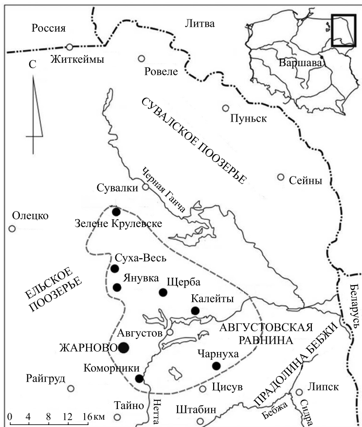
Рис. 1. Местонахождения (закрашенные пунсоны) озерных отложений августовского интергляциала (по [3])
