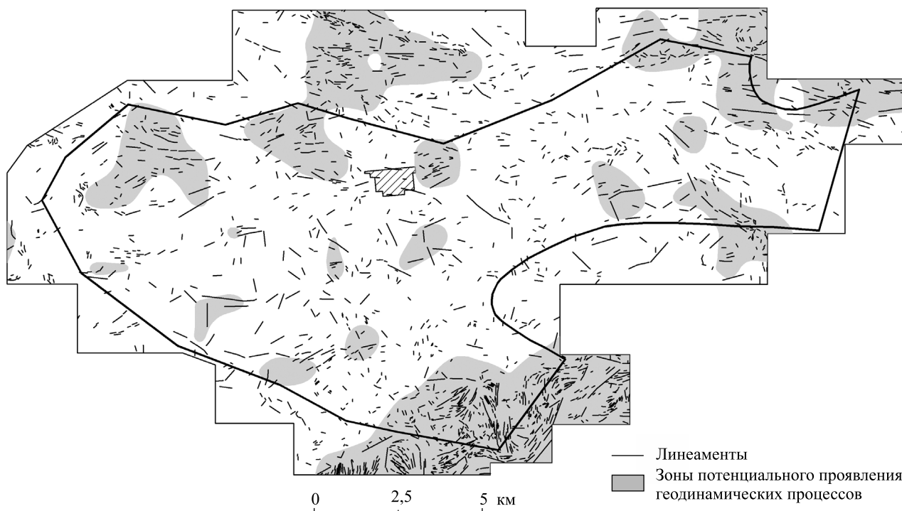
Рис. 2. Поле линеаментов в пределах северного участка Петриковского месторождения
