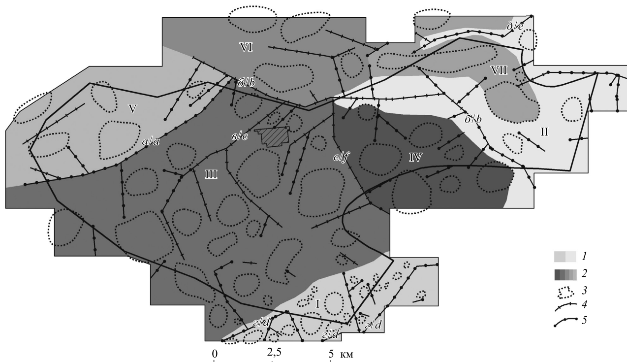
Рис. 4. Неогеодинамически активные структуры в пределах северного участка Петриковского месторождения: 1 – региональные отрицательные структуры; 2 – региональные положительные структуры; 3 – локальные положительные структуры. Системы линеаментов: 4 – представляющие собой активизированные фрагменты разломов кристаллического фундамента и осадочного чехла; 5 – проявившиеся на неотектоническом этапе. Неогеодинамически активные структуры: I – Припятская депрессия; II – Бобриковско-Лукичская депрессия; III – Петриковский купол; IV – Новоселкинский купол; V – Белолесненский купол; VI – Сметанинский купол; VII – Муляровский купол. Линеаменты: а – Железницкий; б – Бобриковский; в – Первомайский; г – Припятский; д – Лукичский; е – Белановичский
