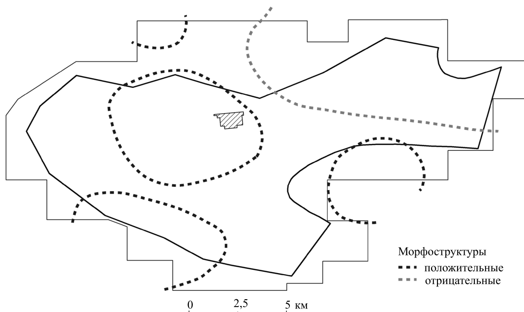
Рис. 3. Морфоструктуры в пределах северного участка Петриковского месторождения
