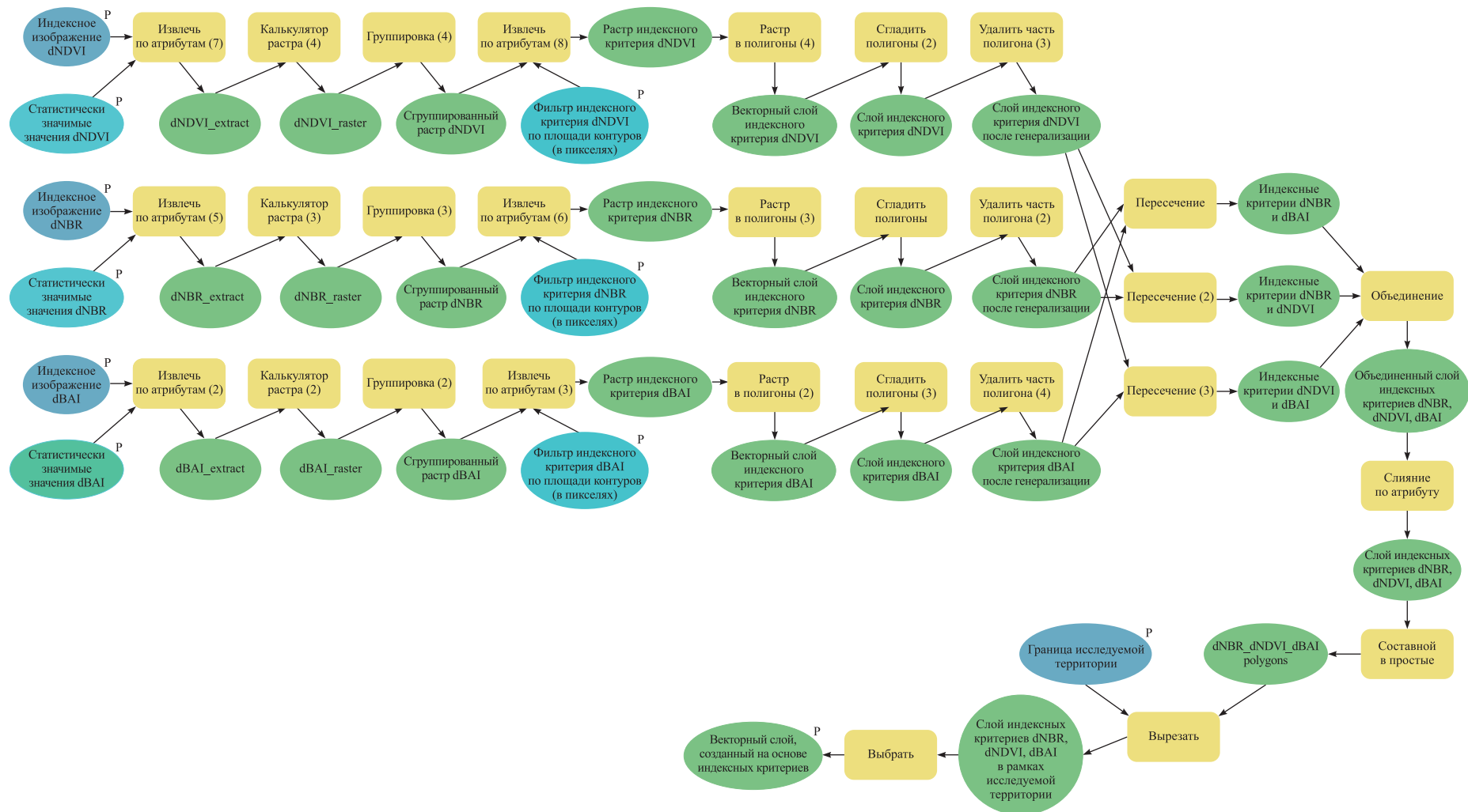
Рис. 2. Модель геообработки для предварительного определения выгоревшей территории на основе индексных критериев (dNBR, dNDVI, dBAI)
