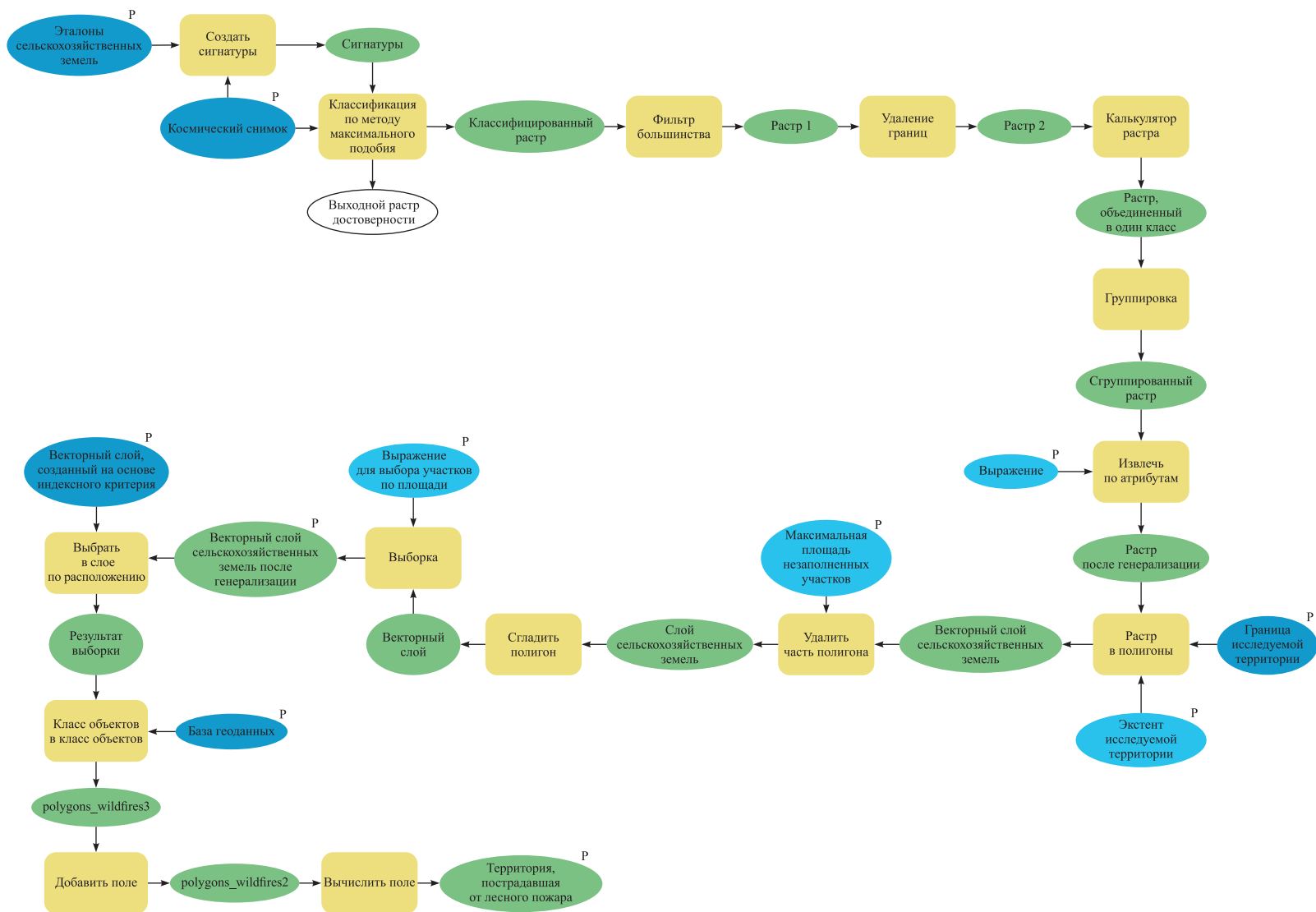
Рис. 3. Модель геообработки для уточнения идентификации лесного пожара (по данным индексных критериев) на основе дешифрирования сельскохозяйственных земель
