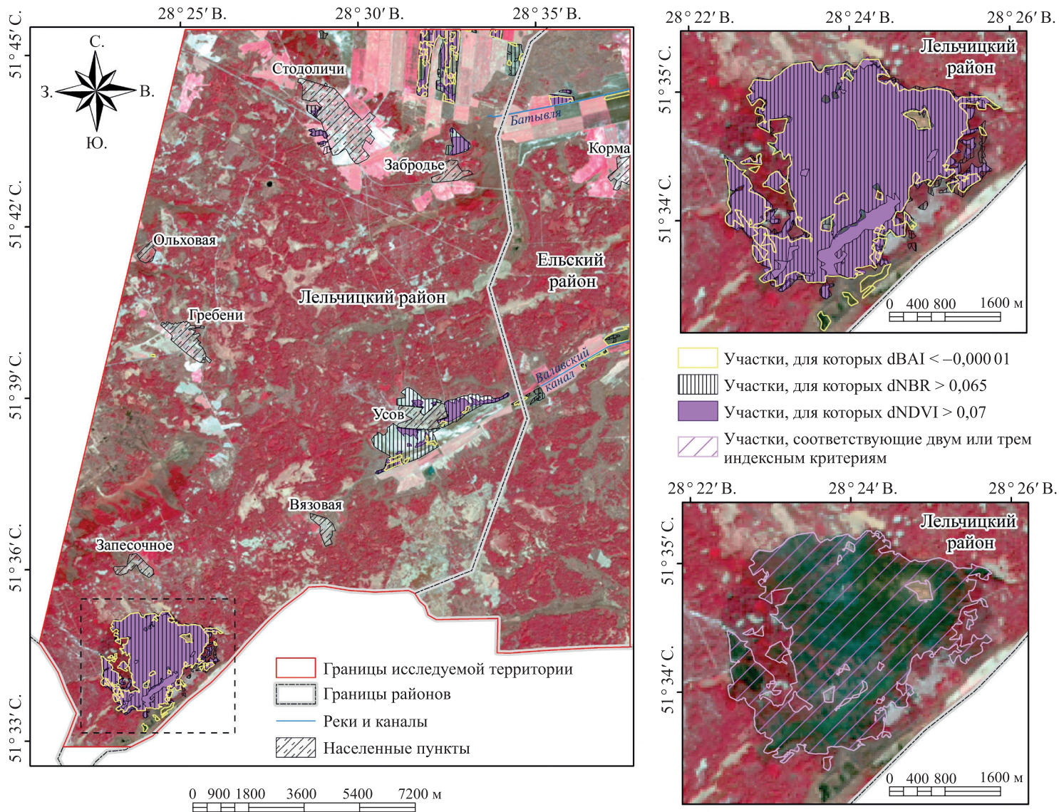
Рис. 4. Карта расположения участков, выбранных на основе разницы индексов NBR, NDVI, BAI за период с 25 марта по 10 апреля 2020 г. по космическим снимкам «Landsat-8»
