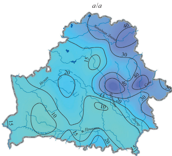
Рис. 3. Распределение наибольших расходов воды весеннего половодья (а) и пространственное распределение трендов максимальных расходов воды весеннего половодья с 1945 по 2020 г. (б), \text{м}^3/\text{с}
