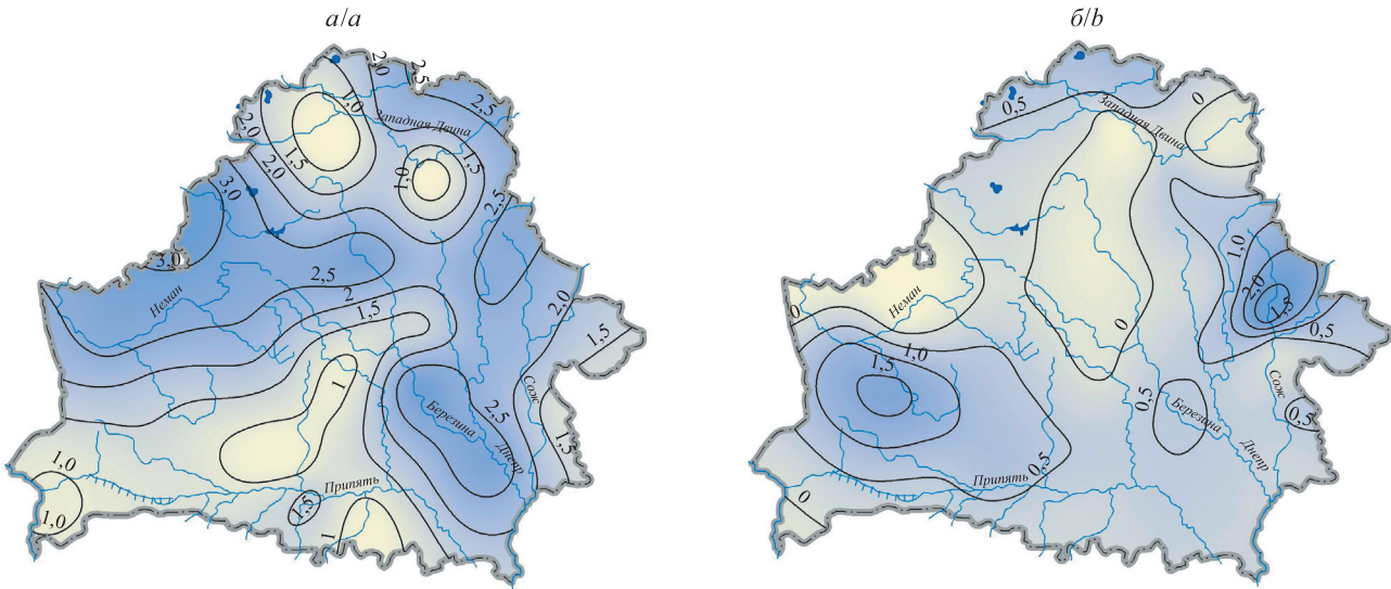
Рис. 4. Распределение наименьших расходов воды летне-осенней межени (а) и пространственное распределение трендов минимальных расходов воды летне-осенней межени с 1945 по 2020 г. (б), \text{m}^3/\text{s}
