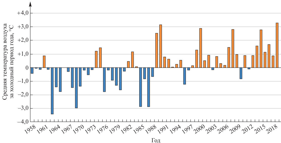
Рис. 3. Средняя температура воздуха за холодный период года с 1958 по 2019 г.
