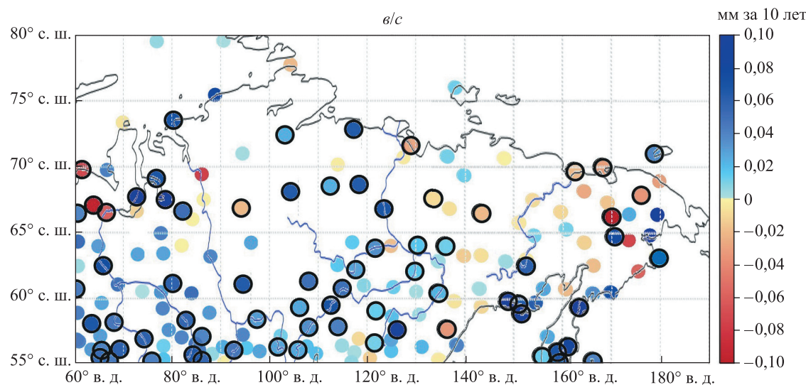
Рис. 2. Многолетние тренды осадков: a – среднее значение; b – количество дней без осадков; c – процентиль 95 %. Точки, имеющие контур, являются значимыми трендами
