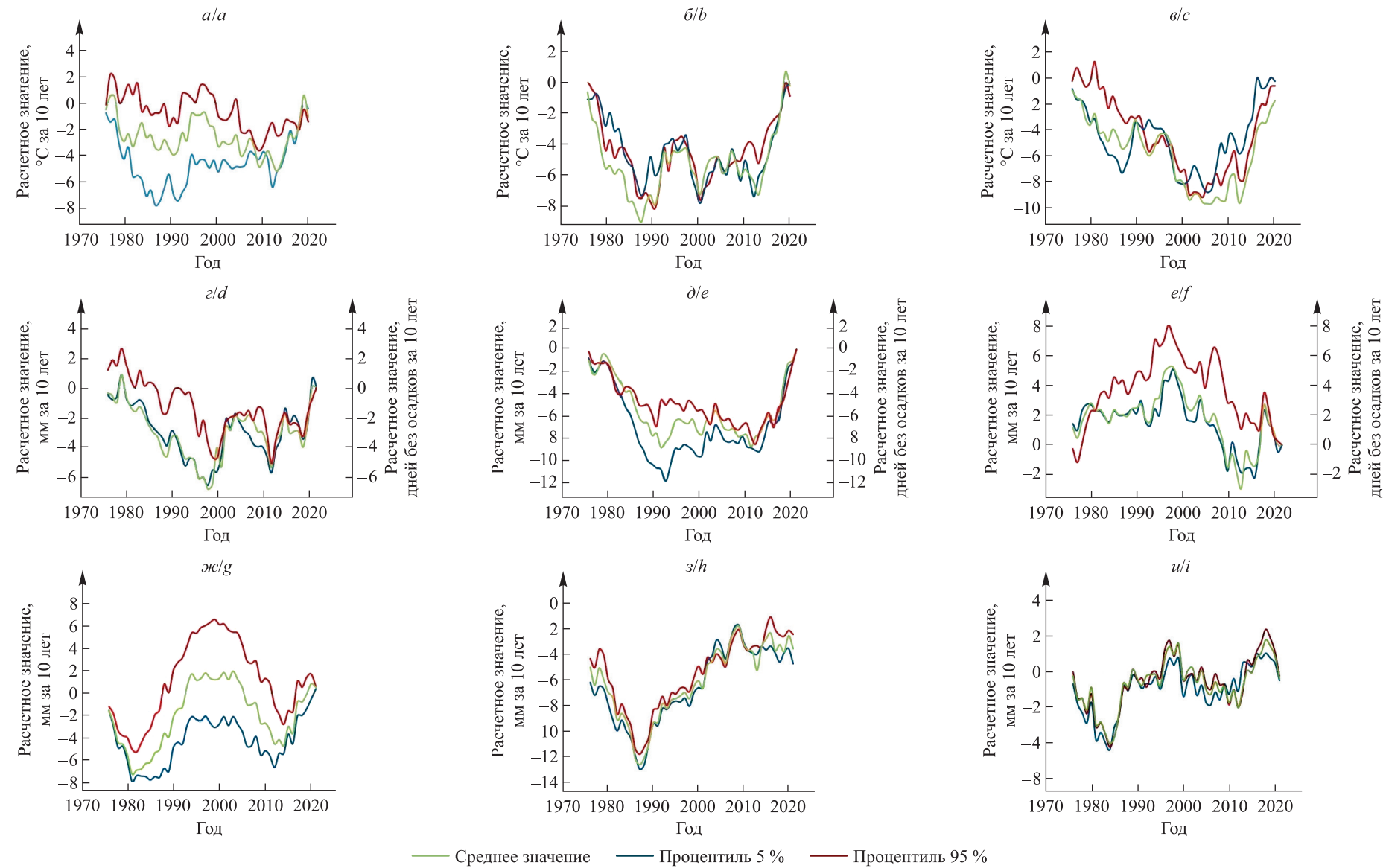
Рис. 4. Интегральные кривые температуры воздуха ( а – в ), осадков и количества дней без осадков ( г – е ), толщины снежного покрова ( ж – и ) в Западной ( а, г, ж ), Центральной ( б, д, з ) и Восточной ( в, е, и ) Сибири (метеорологические станции Толька, Ербогачён и Оймякон)
