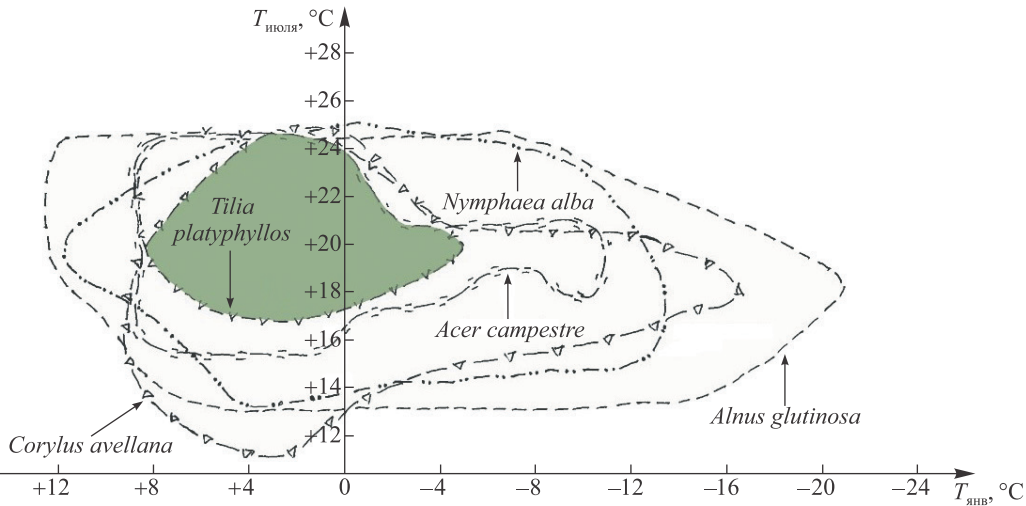
Рис. 2. Реконструкция палеотемпературных показателей для атлантического периода голоцена разреза «Брод» на р. Западной Березине
