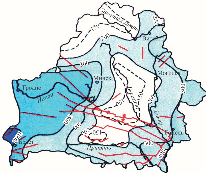
Рис. 6. Схема глубины залегания подошвы пресных вод в Беларуси. Звездочками отмечены отдельные аномалии разгрузки глубинных минерализованных вод над разломами. Источник: [5], с изменениями
