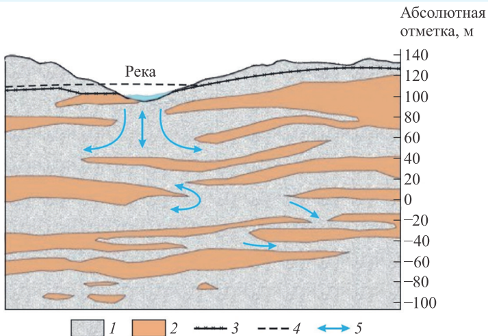
Рис. 8. Пример, поясняющий строение верхней части геологического разреза в зоне распространения пресных вод с гидрогеологическими окнами, соединяющими водоносные горизонты: 1 – водоносные отложения; 2 – относительные водоупоры; 3 – нормальное положение зеркала грунтовых вод; 4 – положение зеркала грунтовых вод в периоды половодья; 5 – направления фильтрации воды.
