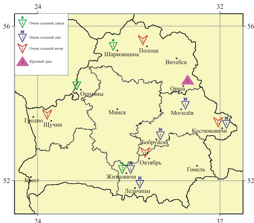
Рис. 7. Повторяемость ОЯП, вызванных западными циклонами за период 1995–2015 гг.
