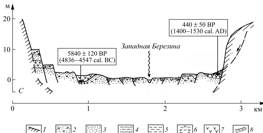
Рис. 9. Схематический геологический профиль через долину р. Западной Березины в пределах Ошмянской конечной моренной гряды: 1 – отложения коренных склонов; 2 – песок с гравием; 3 – песок; 4 – пылеватый песок и супесь; 5 – суглинок; 6 – торфяной ил; 7 – торф; 8 – отложения делювиальных конусов выноса. Источник: [8]
