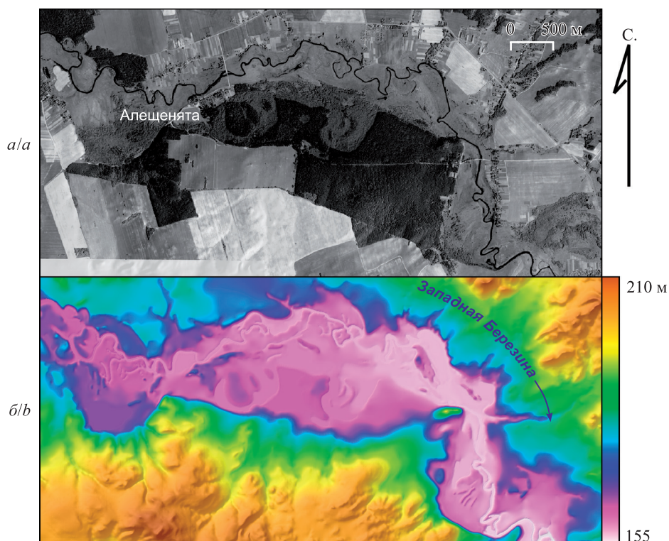
Рис. 8. Участок долины р. Западной Березины у д. Алещенята Воложинского района по материалам АФС: а – фрагмент ортофотоплана; б – матрица высот
