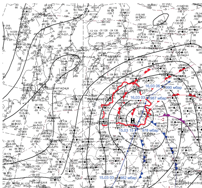
Рис. 4. Приземная карта за 15 марта 2013 г. (15 UTC) – выход южного циклона, сопровождавшегося сильными снегопадами (указана траектория циклона за период 15–16 марта 2013 г.)
