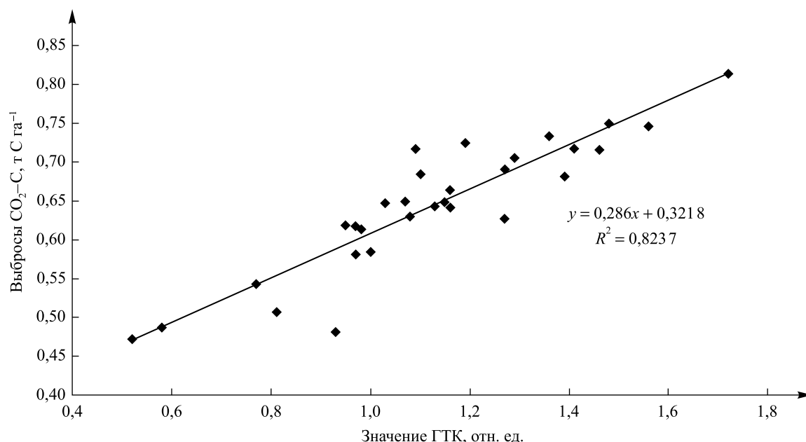
Рис. 5. Зависимость выбросов углерода \text{CO}_2\text{-C} на поле с озимой пшеницей в десятипольном севообороте от средних за вегетационный период значений GTK (вариант без внесения удобрений, климатический сценарий RCP4.5)
