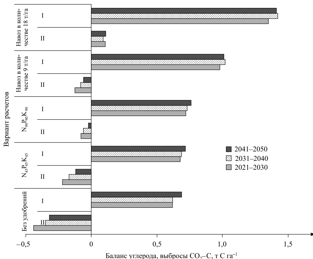
Рис. 7. Динамика ожидаемых средних по десятилетиям годовых значений баланса углерода и выбросов углерода \text{CO}_2\text{--C} на отдельном поле севооборота при разных вариантах внесения удобрений (климатический сценарий RCP8.5): I – выбросы \text{CO}_2\text{--C} ; II – баланс углерода
