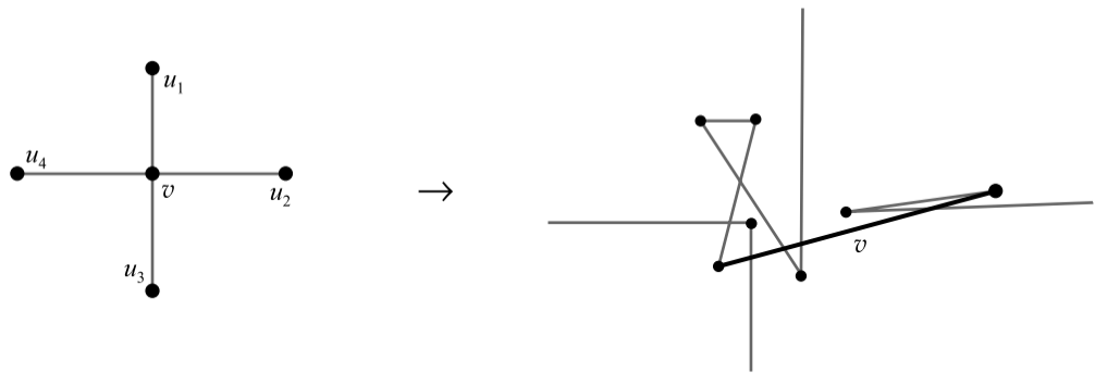
Рис. 7. Преобразование вершины степени 4 Fig. 7. Transformation of vertex with degree 4
