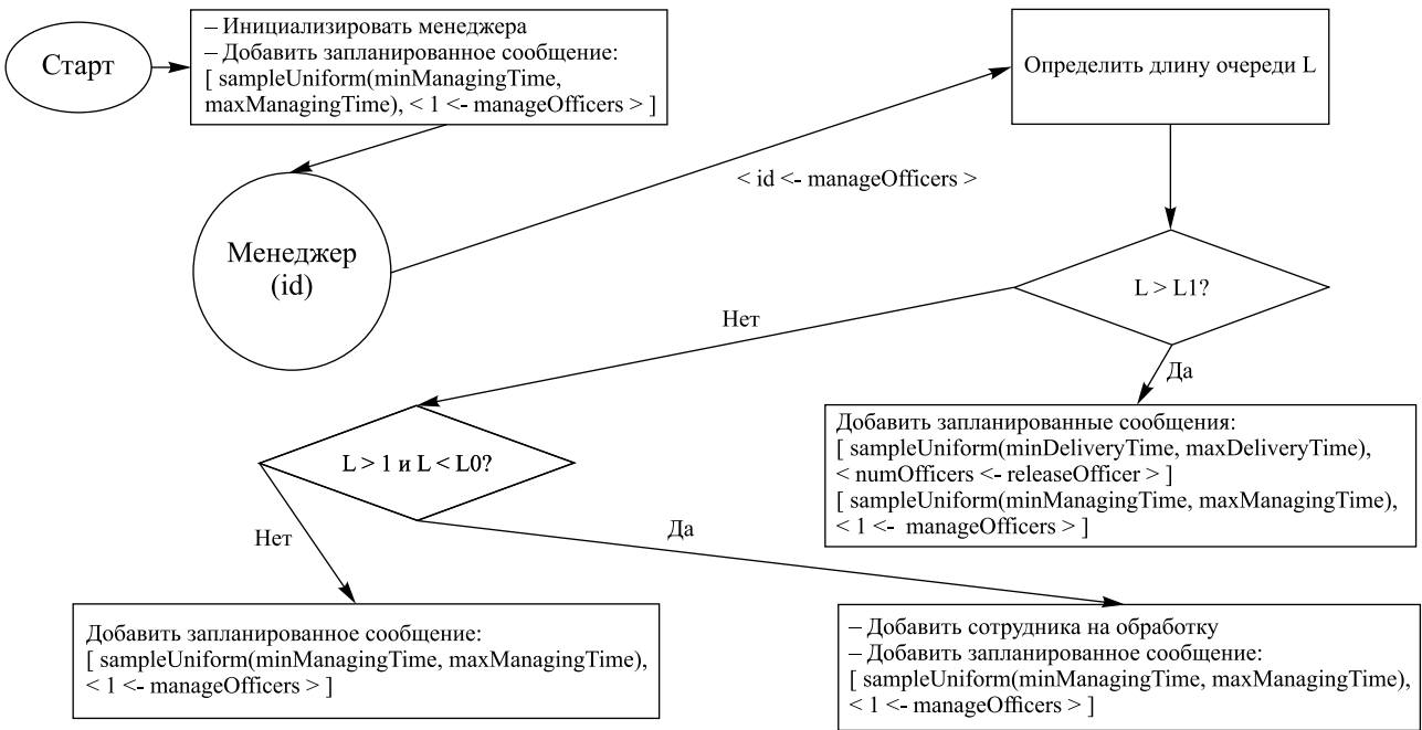
Рис. 8. Алгоритм менеджера
