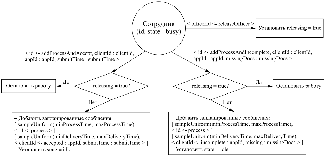
Рис. 9. Алгоритм сотрудника при наличии менеджера
