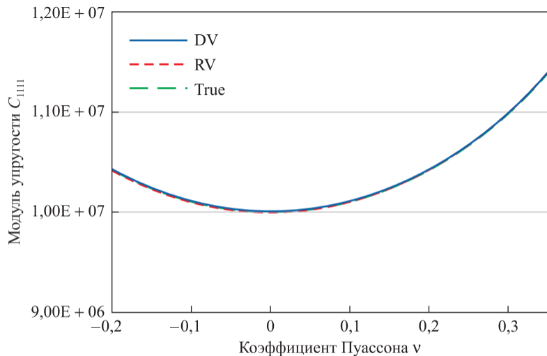
Рис. 5. Восстановление модуля упругости C_{1111} при различных коэффициентах Пуассона
