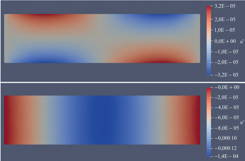
Рис. 8. Эксперимент 2. Визуализация решения модели DV
