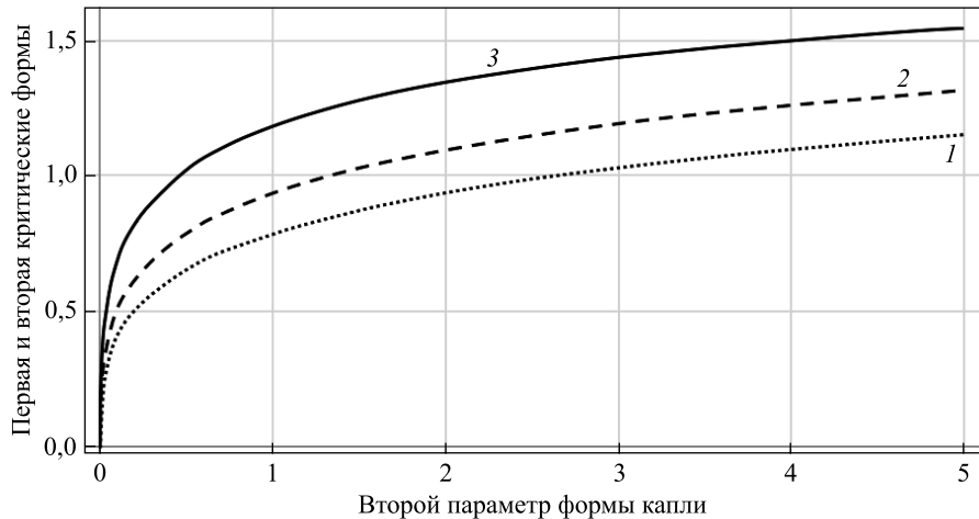
Рис. 3. Зависимость критических значений второго параметра формы капли от первого параметра: 1 – первая критическая форма при краевом угле 90^\circ ; 2 – первая критическая форма при краевом угле 180^\circ ; 3 – вторая критическая форма
