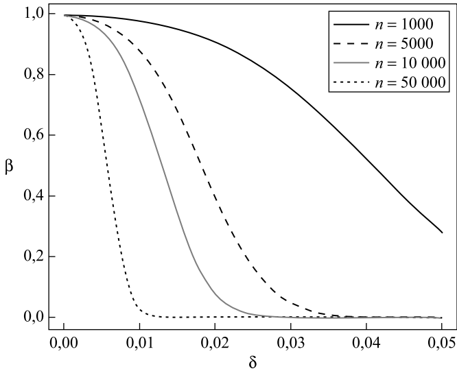
Рис. 2. Зависимость вероятности ошибки второго рода \beta от параметра \delta для теста Monobit (МДРН(1)):
