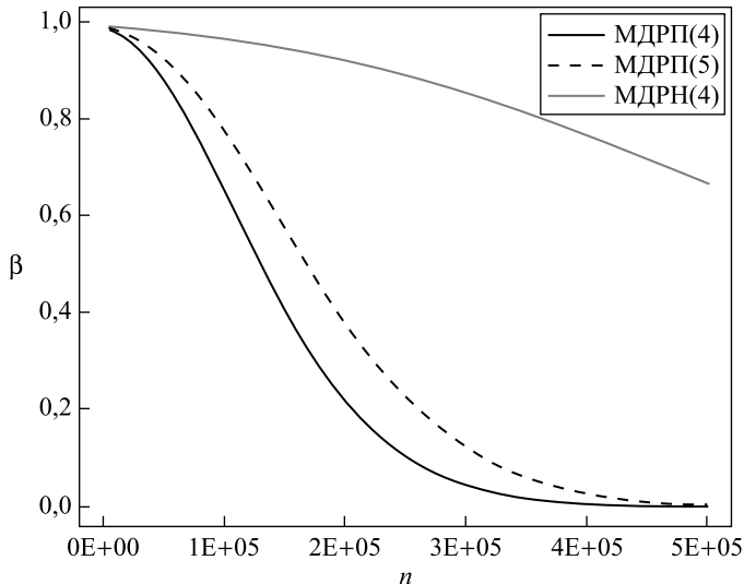
Рис. 5. Зависимость вероятности ошибки второго рода \beta от размера выборки n для тестов МДРП(4), МДРП(5) и МДРН(4): H_1 = MC(3, 1) , \alpha = 0,01 , \delta = 0,005
