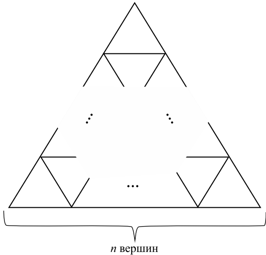
Рис. 1. Треугольная решетка
