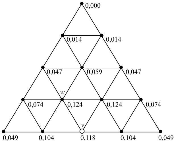
Рис. 2. Вероятности достижения каждой из вершин блужданием длины 3
