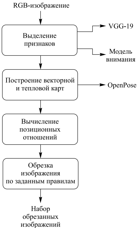
Рис. 2. Алгоритм Smart Cropping
