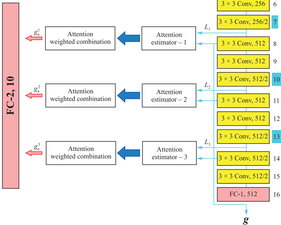
Рис. 5. Архитектура модели внимания
