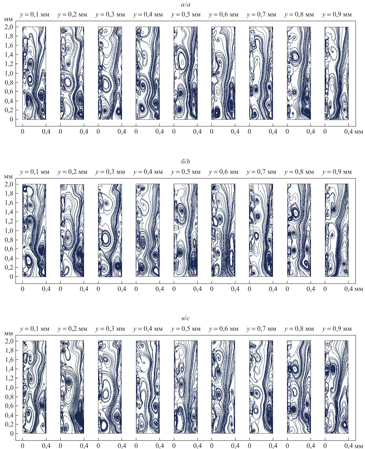
Рис. 2. Линии тока жидкости в сечениях y = 0,1; 0,2; 0,3; 0,4; 0,5; 0,6; 0,7; 0,8; 0,9 мм для трехмерной модели в момент времени 108 с (а), 108,25 с (б), 108,5 с (в)
