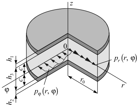
Рис. 1. Расчетная схема трехслойной пластины
