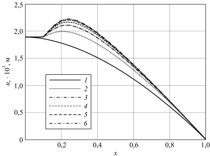
Рис. 2. Сходимость итерационного метода при \varphi = 0 , T = 293 \text{ K} : 1, 2, 3, 4, 5, 6 – номер итерации
