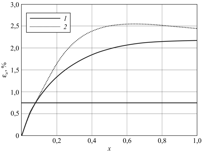
Рис. 3. Интенсивность деформаций \varepsilon_u при \varphi = 0 : 1 – упругая пластина; 2 – упругопластическая пластина
