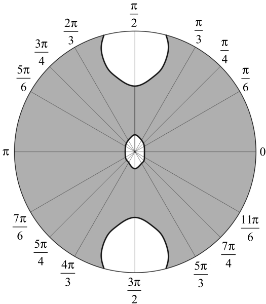
Рис. 4. Распределение областей пластичности и физической нелинейности (серый цвет) в зависимости от окружной координаты
