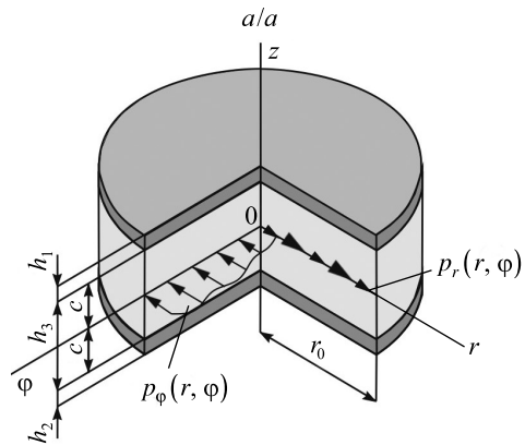
Рис. 1. Расчетная схема трехслойной пластины при нагружении в своей плоскости
