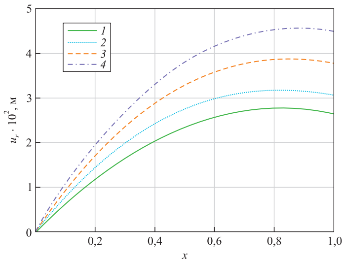
Рис. 3. Радиальные перемещения u_r в трехслойной пластине при различных температурах: 1 – упругая пластина при T = 293 К; 2, 3, 4 – упругопластическая пластина при T = 293 К, T = 373 К, T = 473 К соответственно
